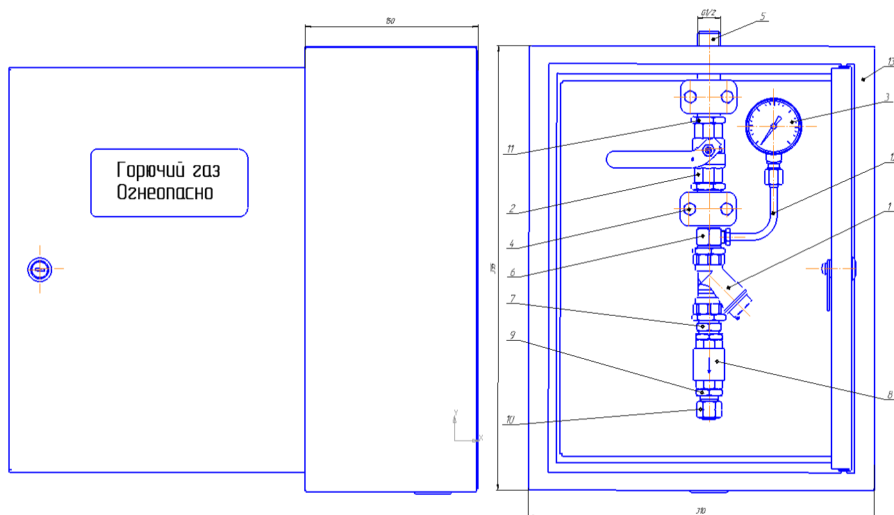
Рис. 1. Пост газоразборный ППГ-10-3
